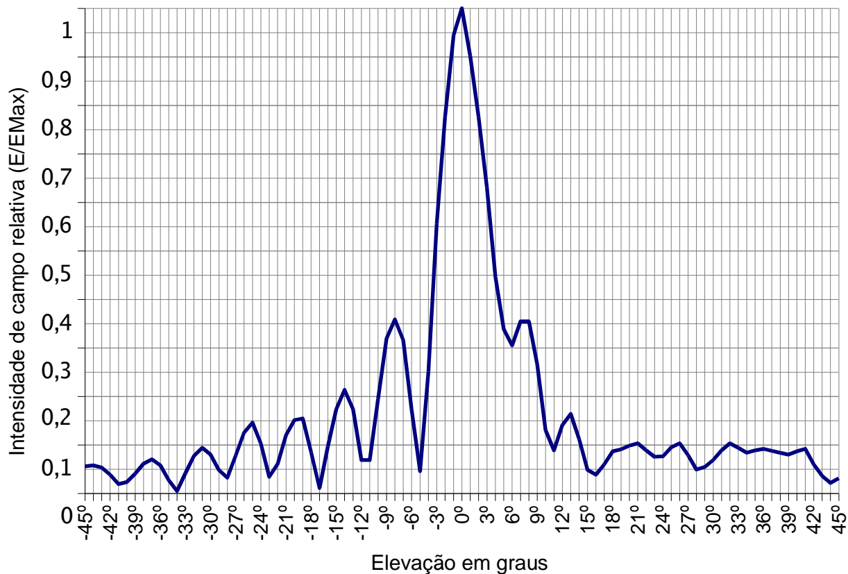
Omnidirecional para WLL Diagrama de elevação para 15dBi
